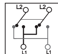
Moduł łączytki krzyżowego
